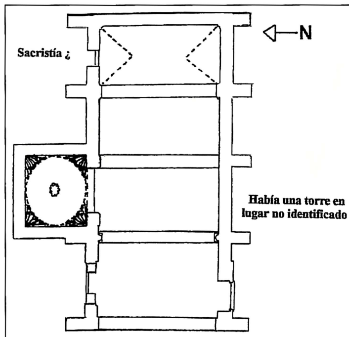
Cenizate. Iglesia Parroquial. Planta hipotética que podría tener la iglesia a finales del primer tercio del siglo XVII.
