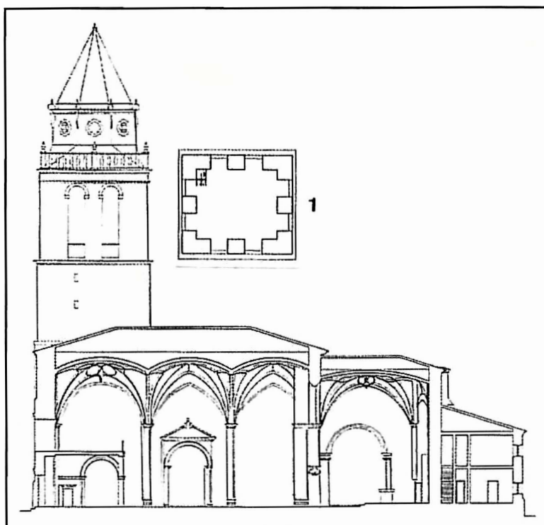
Mahora. Parroquia de Santa María de la Asunción. Sección longitudinal. 1: planta del cuerpo de campanas de la torre.
