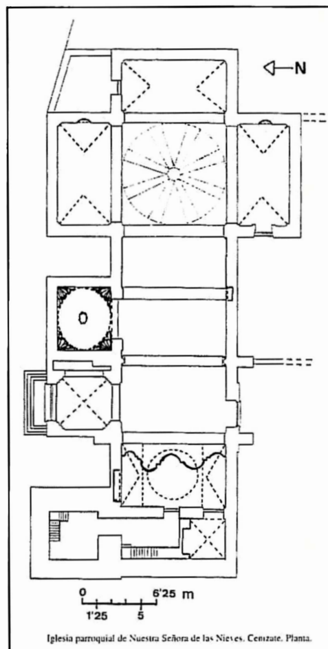
Cenizate. Iglesia Parroquial. Planta.
