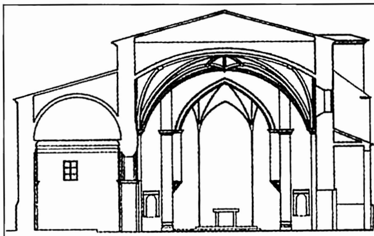
Mahora. Parroquia de Santa María de la Asunción. Sección transversal.
