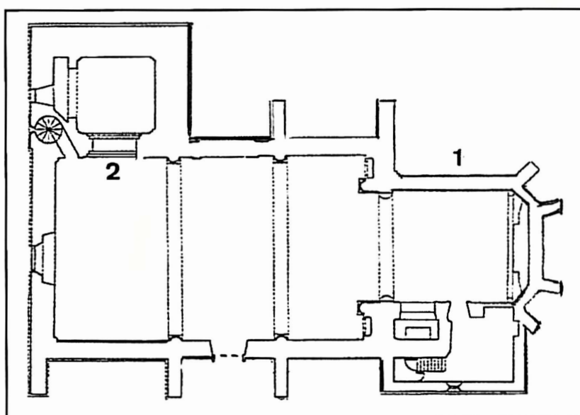
Mahora. Parroquia de Santa María de la Asunción. Planta hipotética de la iglesia a finales del primer tercio del siglo XVI. 1: es probable que hubiera en ese lugar una capilla; 2: la capilla tal como hoy puede contemplarse en el interior del cuerpo bajo de la torre se remodeló en el siglo XVIII, pero no sé si el acceso entre este espacio y el tercer tramo de la nave existiría ya en el siglo XVI.
